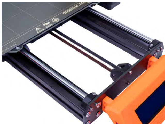
Obr. 47 - Správně napnutý řemen pod vyhřívanou podložkou
