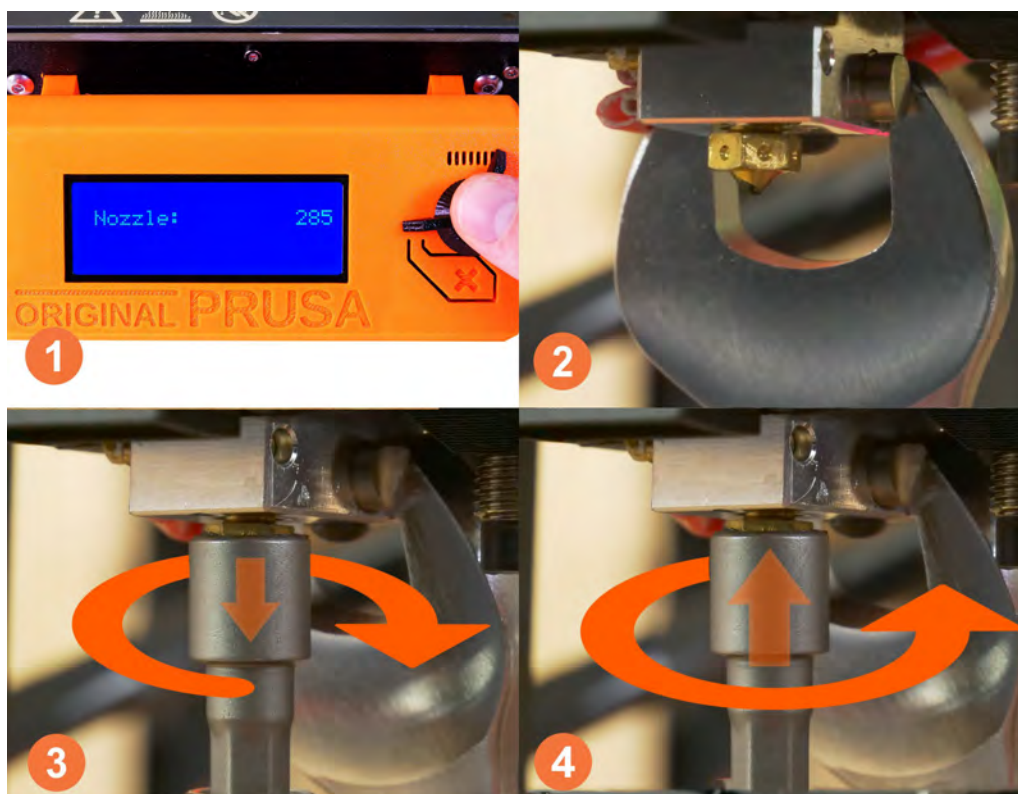
Obr. 42 - Výměna trysky
