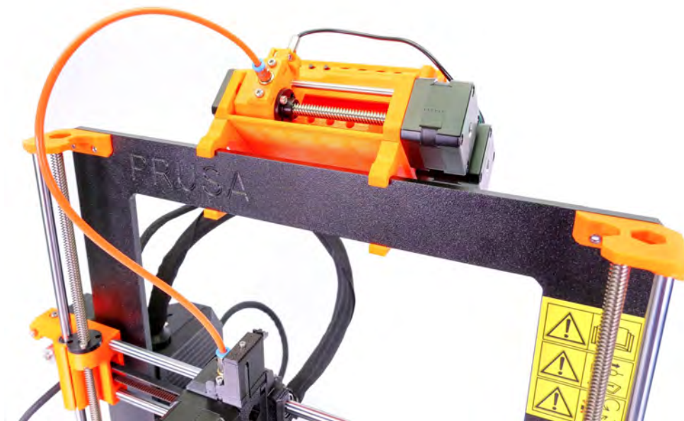
Obr. 23 - Multi Material Upgrade 2S na tiskárně Original Prusa i3 MK3S+
