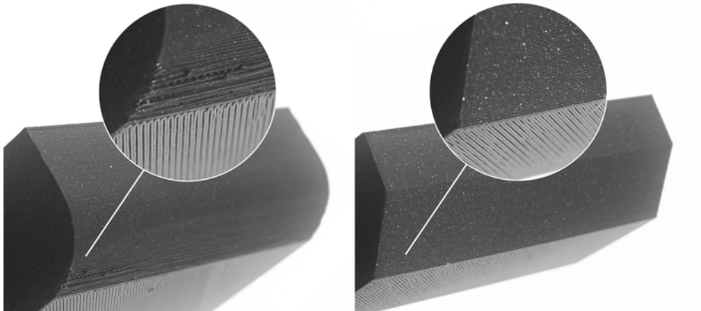
Obr. 28 - Zaoblení (vlevo) vs zkosení (vpravo) hrany
