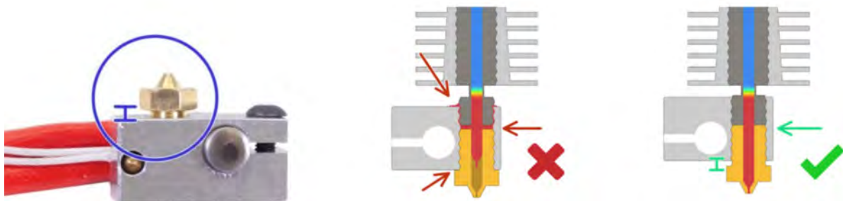
Obr. 41 – Mezera mezi tryskou a topným blokem při plném dotažení
