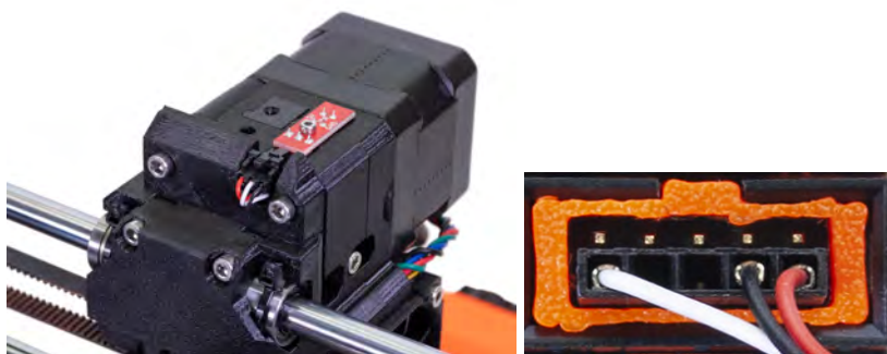
Obr. 38 - Správné usazení a připojení senzoru filamentu
