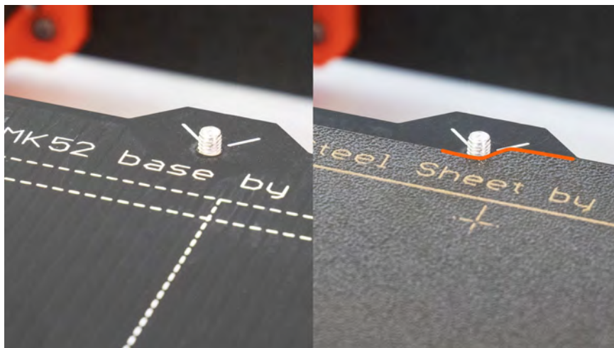
Obr. 5 - Vyhříváná podložka MK52 a tiskový plát se zrnitým práškovým PEI povrchem
