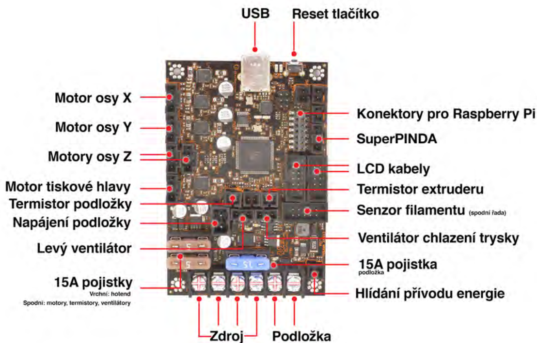
Obr. 46 - Správné zapojení konektorů
