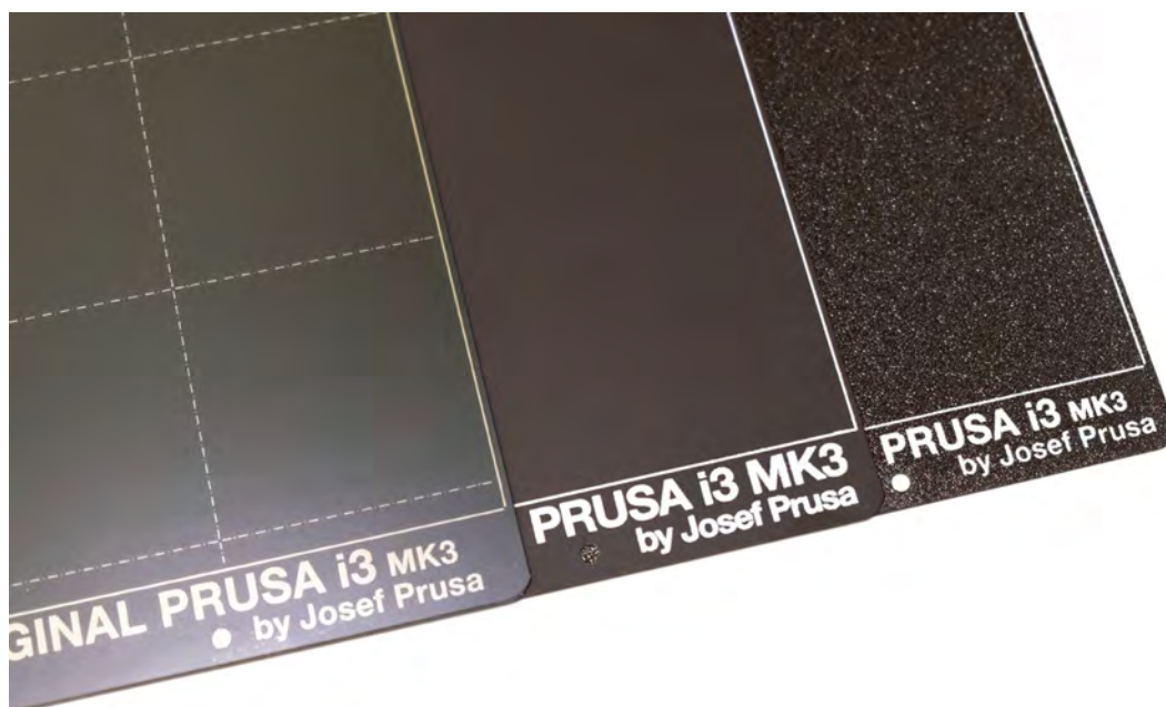
Obr. 6 - Ocelové tiskové pláty - hladký PEI povrch, saténový práškový povrch a zrnitý práškový PEI povrch
