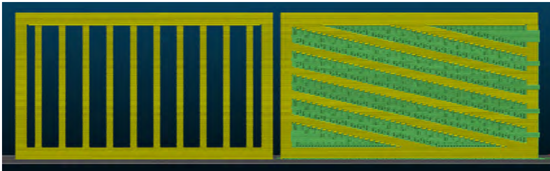
Obr. 27 - Model tisknutelný bez podpor vs model vyžadující velké množství podpor
