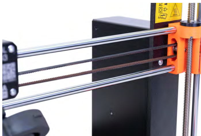
Obr. 48 - Správně napnutý řemen u tiskové hlavy
